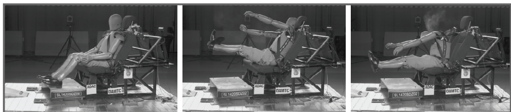
Abbildung 5: Schlittenversuch Nr. 8 in einer leicht gedrehten (15°) Sitzposition
