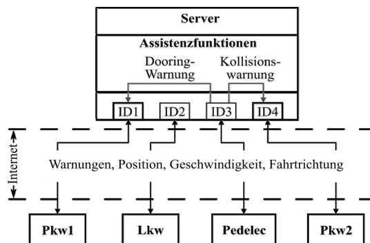
Abbildung 37: Konzeptübersicht Demonstrator Dooring- und Kollisionswarnung
